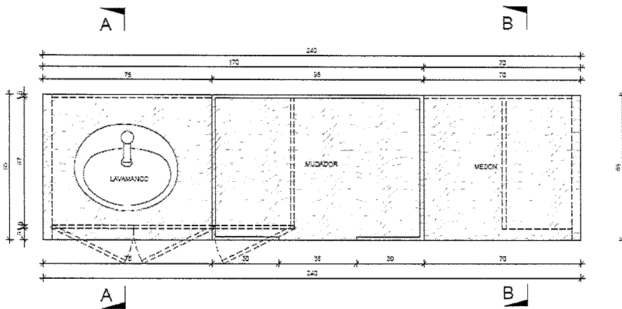
PLANTA GENERAL ESC 1:10
