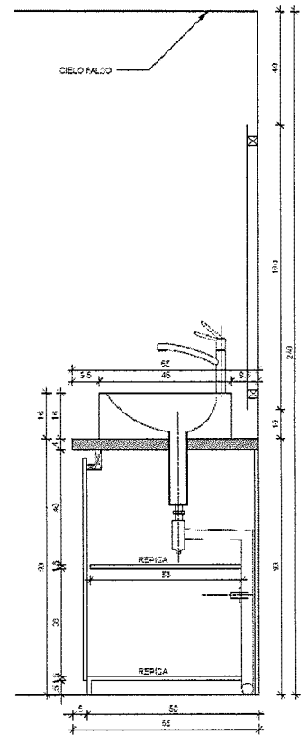
CORTE A-A ESC 1:10
