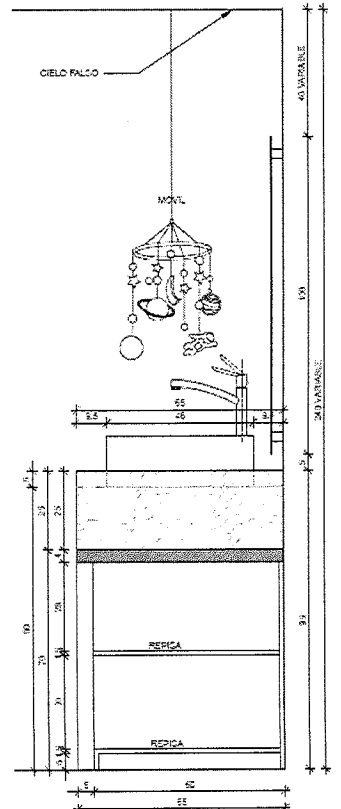
CORTE B-B ESC 1:10
