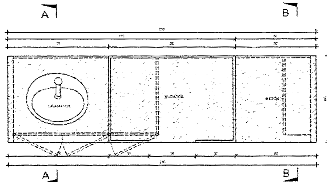
PLANTA MUEBLE MUDADOR EN OBRA / SALA DE LACTANCIA / ESC 1:10'
