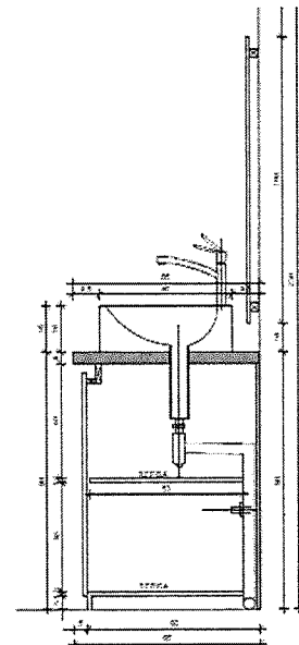
CORTA A-A / ESC 1:10'
