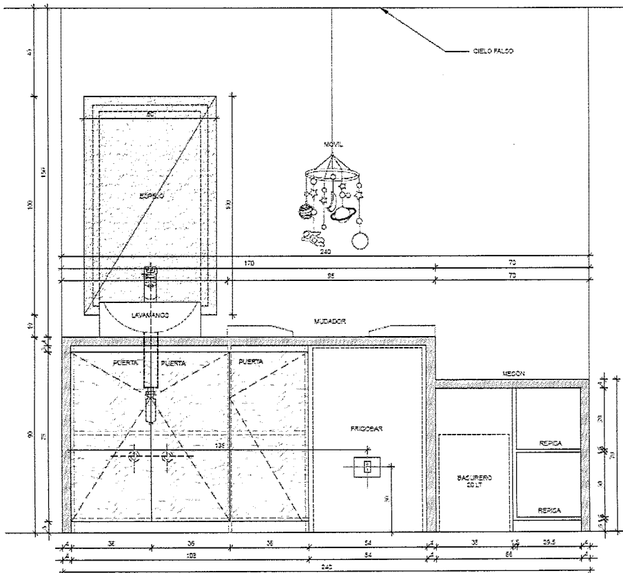
ELEVACIÓN ESC 1:10
