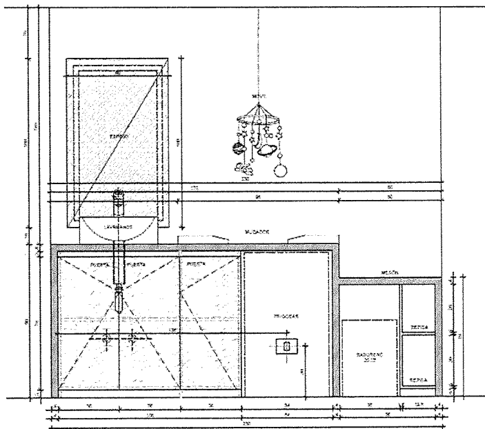
ELEVACION MUEBLE MUDADOR / ESC 1:10'
