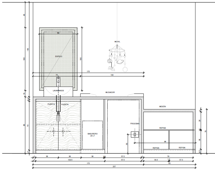
ELEVACIÓN MUEBLE MUDADOR / ESC 1:10/
