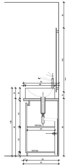
CORTA A-A / ESC 1:10/
