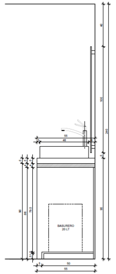
CORTA B-B / ESC 1:10/
