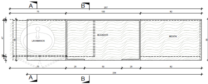
PLANTA MUEBLE MUDADOR EN OBRA / SALA DE LACTANCIA / ESC 1:10/
