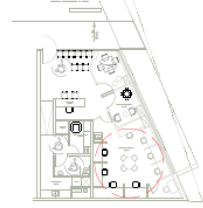
PLANTA UBICACIÓN MUEBLE MUDADOR EN OBRA / SALA DE LACTANCIA / ESC 1:10/
