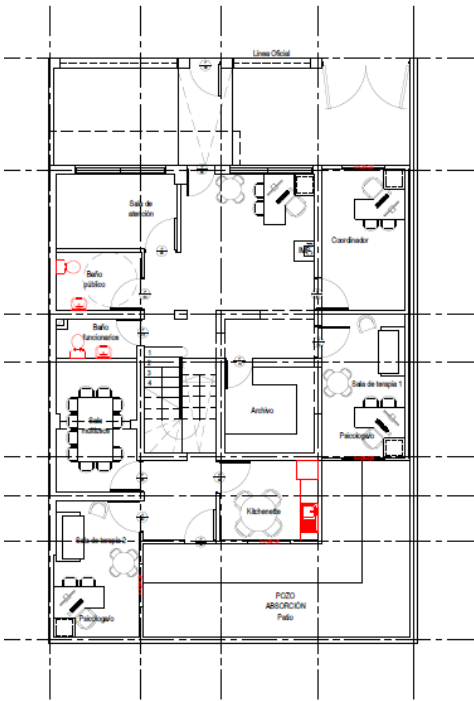
PLANTA ARQUITECTURA 1º PISO asc. 150 108,78 m 2 Construido
