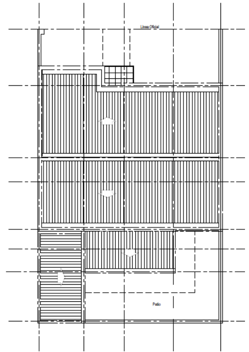
PLANTA CUBIERTA asc. 150
