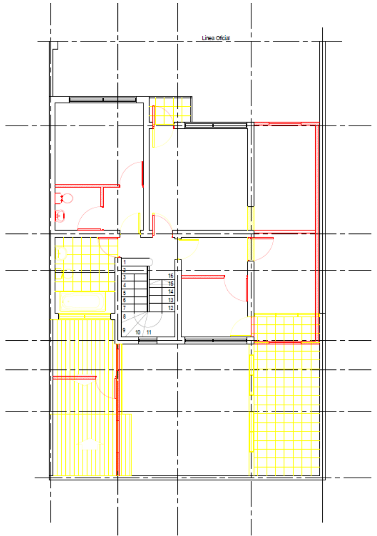
PLANTA ARQUITECTURA 2º PISO esc. 1:50 102,41 m2 Construidos
