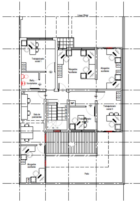
PLANTA ARQUITECTURA 2º PISO asc. 150 102,41 m 2 Construido
